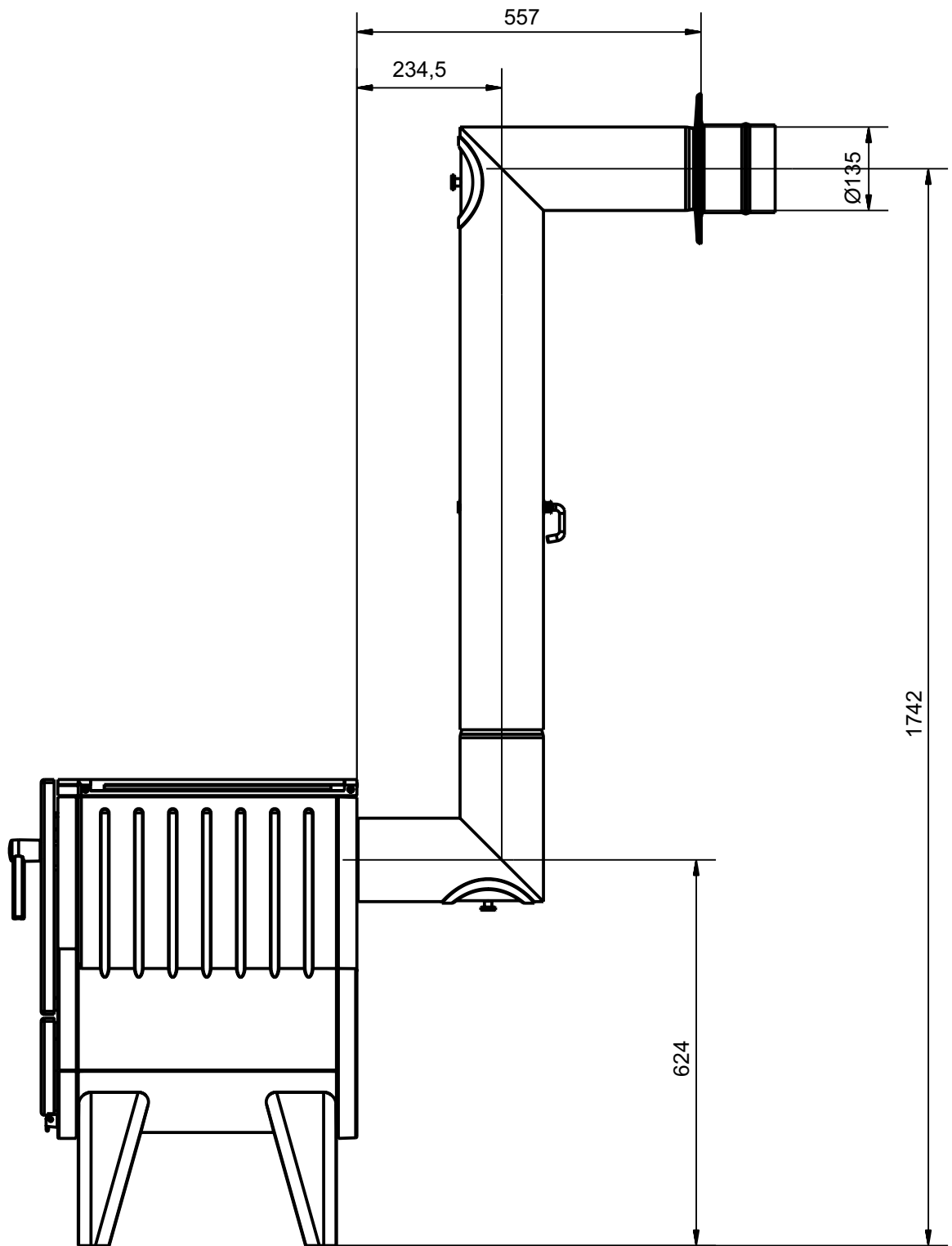
Iron-Dog 03 Rauchrohr vertikal
