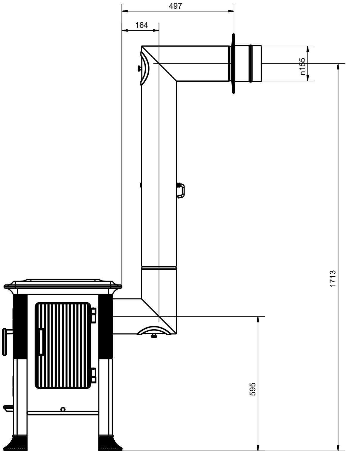
Iron-Dog 04 Rauchrohr vertikal
